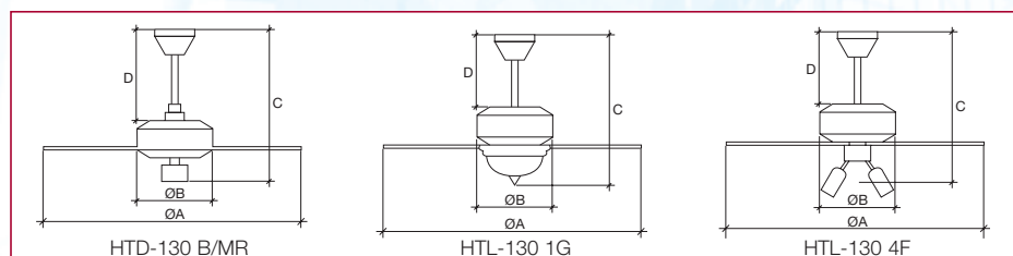
Mod. HTD-130 MR Omkeerbare vleugel Donker bruin Licht bruin
