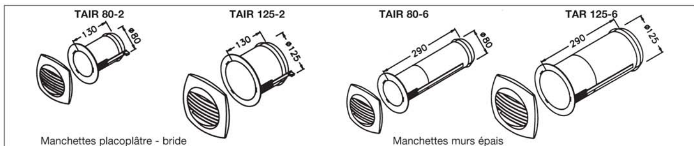
Manchettes placoplâtre - bride
